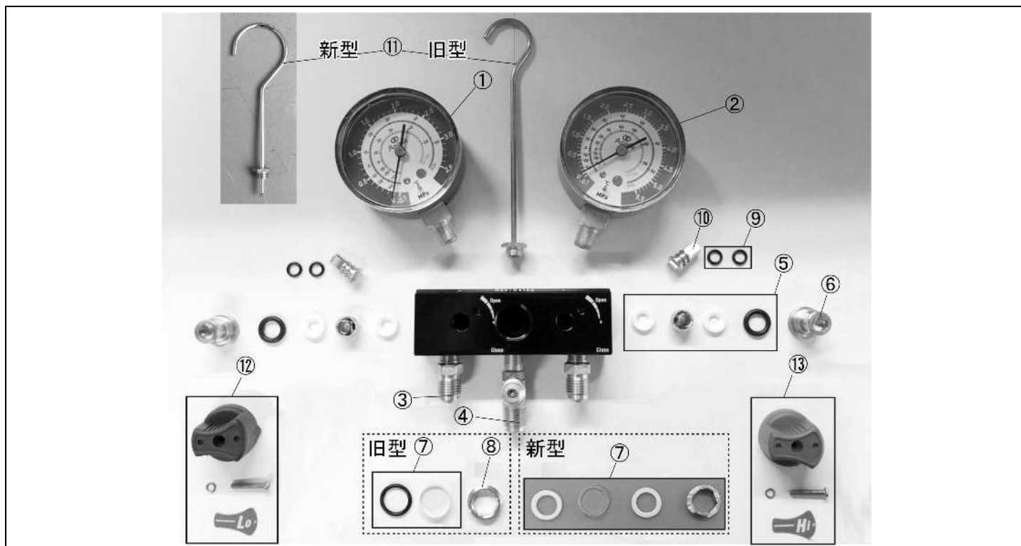
ボールバルブ式 Mini マニホールド R32,410A (AI186)
