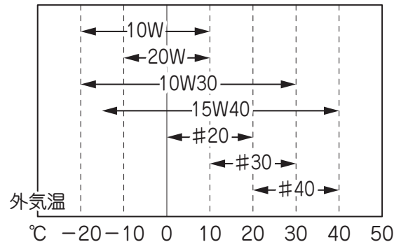
潤滑油粘度表 (SAE 分類)
